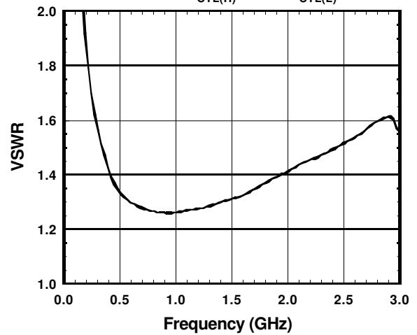
VSWR(P4) vs. Frequency
