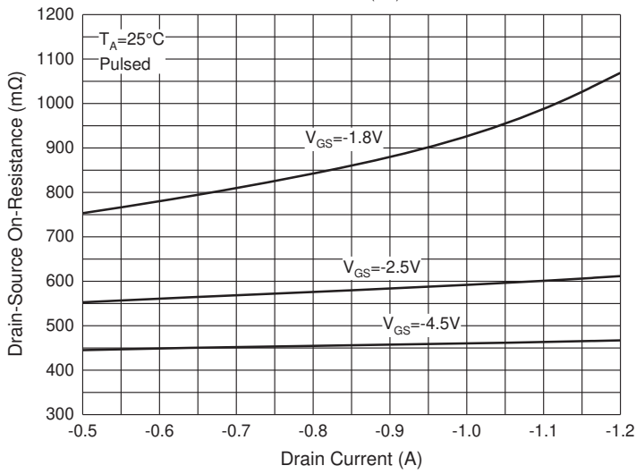
Fig. 9 - R_{DS(ON)} - I_D
