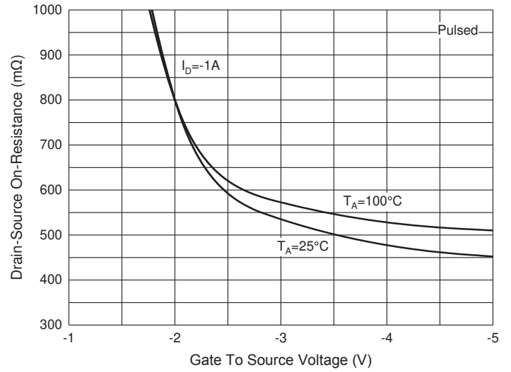
Fig. 10 - R_{DS(ON)} - V_{GS}
