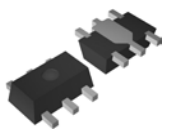
SOT-89-5 4.5 x 4.35 x 1.5
