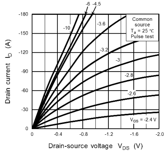
Fig. 8.2 I_D - V_{DS}
