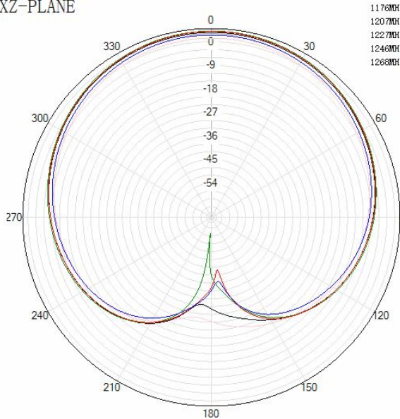
XZ-PLANE
