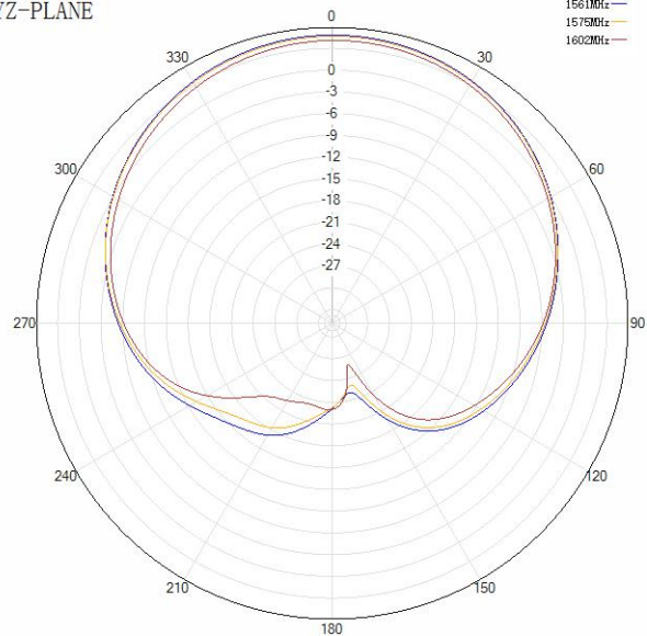
YZ-PLANE
