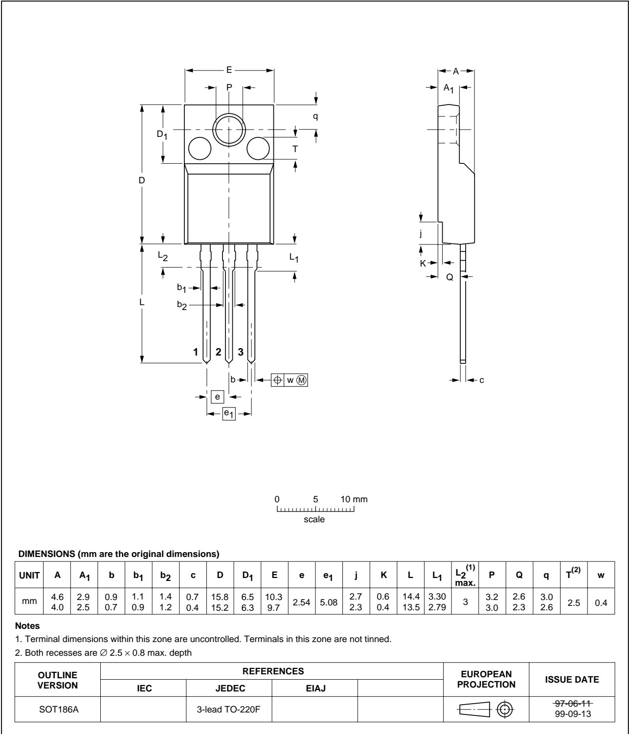
Fig 15. SOT186A.
