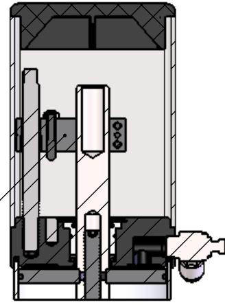
SECTION B-B SCALE 1 : 4
