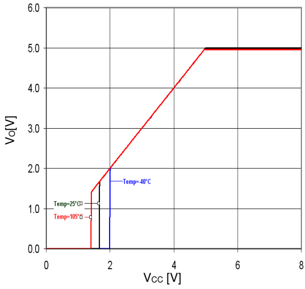
Fig.27 Vcc-Vo (Io=0mA)
