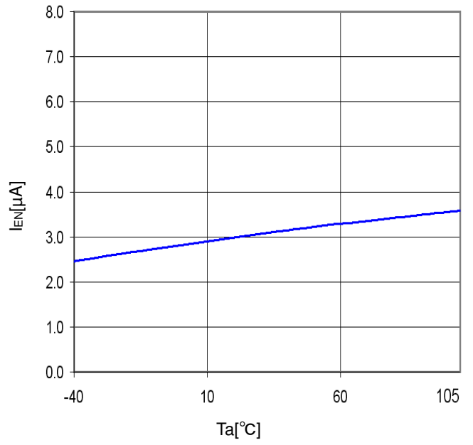
Fig.24 T_a - I_{EN}
