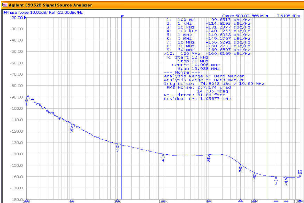
Figure 1. LVPECL Output 500MHz 12kHz-20MHz 82fs
