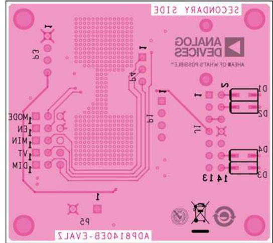
Figure 23. ADP8140EB-EVALZ Bottom Layer
