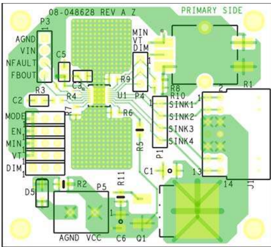
Figure 20. ADP8140EB-EVALZ Top Layer
