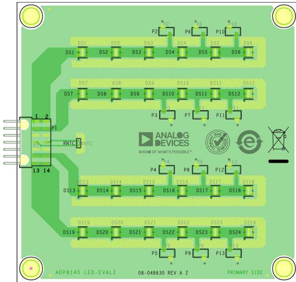
Figure 24. ADP8140 LED-EVALZ Top Layer
