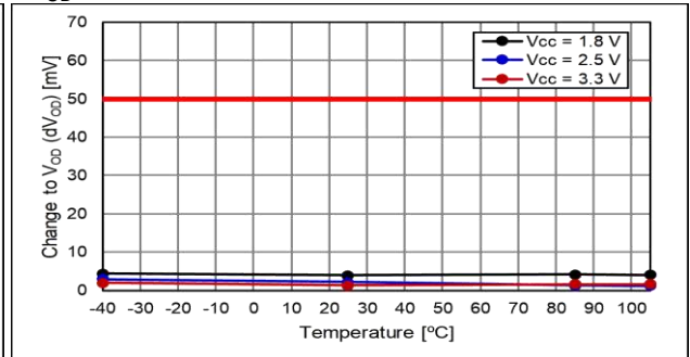
dV OD
