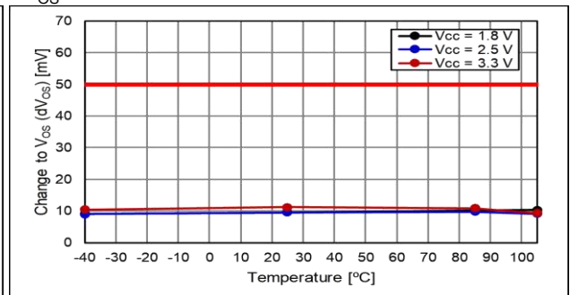
dV OS
