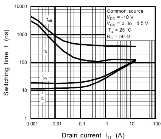
Fig. 7.9 t - I_D
