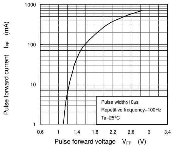
I_{FP} - V_{FP}
