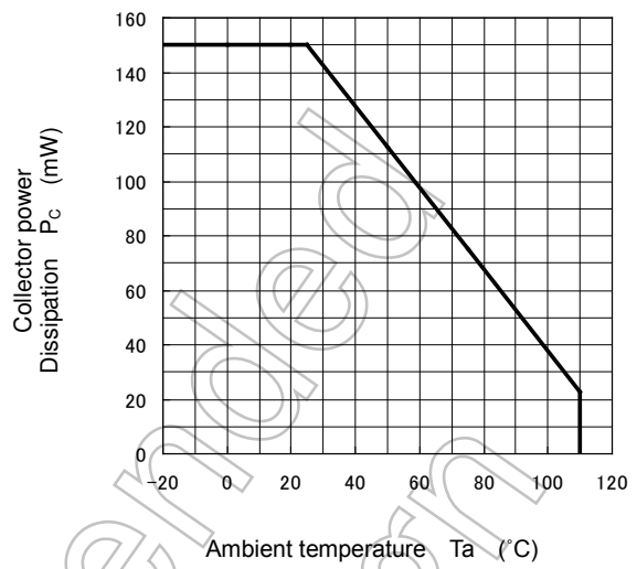
P_C - T_a
