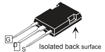
ISOPLUS247™ (IXFR) E153432
