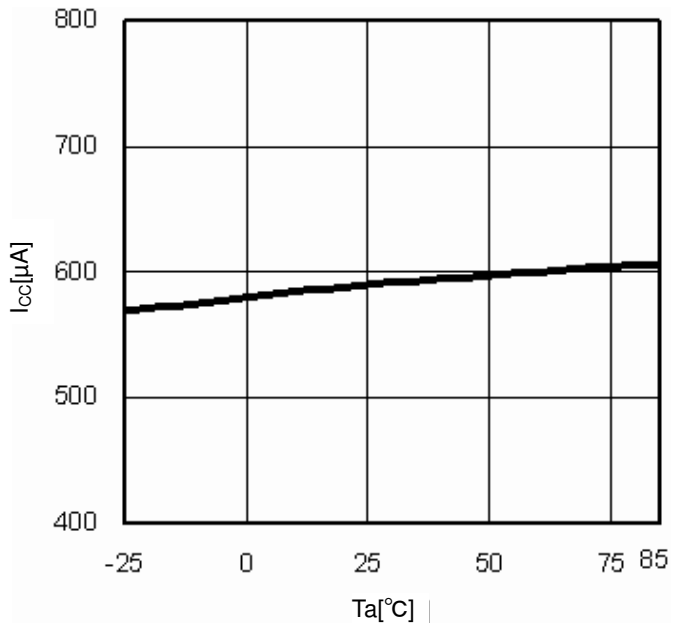
Fig.10 T_a-I_{cc}
