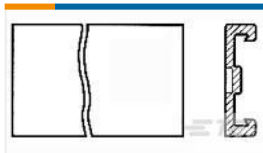
TE Part #640643-5 05P MTA156 COVER F/T
