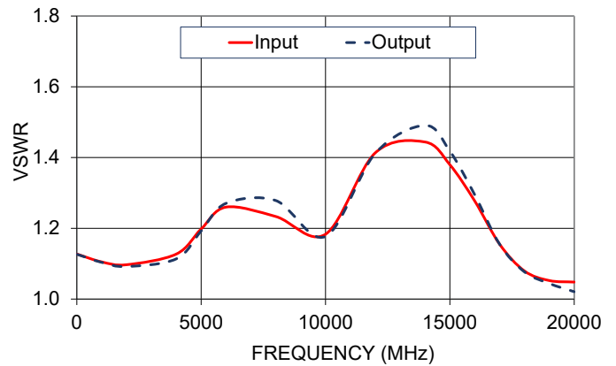
EQY-5-24+ VSWR
