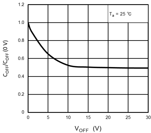
Fig. 12.11 C_{OFF} / C_{OFF} - V_{OFF}
