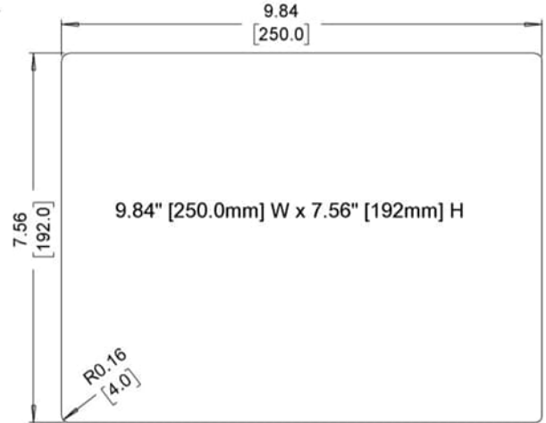
Cutout Dimensions
