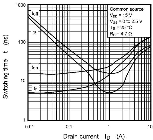
Fig. 8.11 t - I_D
