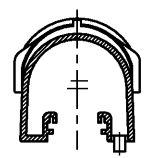
SECTION Schnitt A-A
