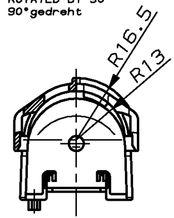
SECTION Schnitt A-A
