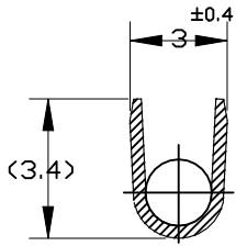
SECT A-A
