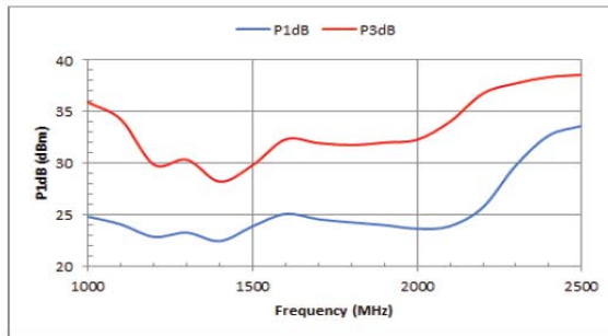
P1dB & P3dB
