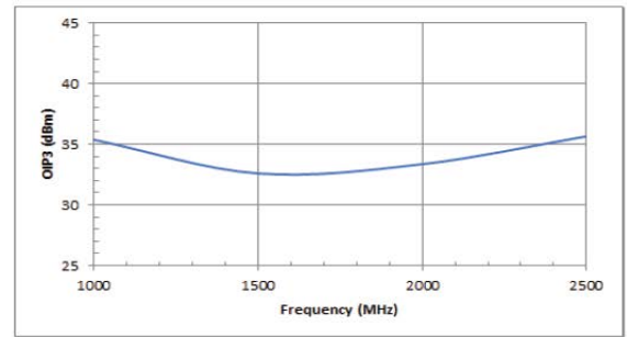
OIP3
