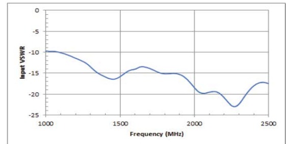
VSWR
