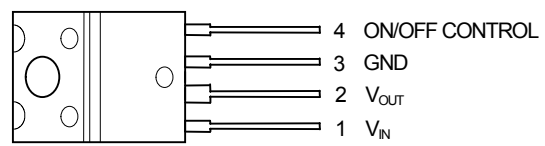
NJM2388F
