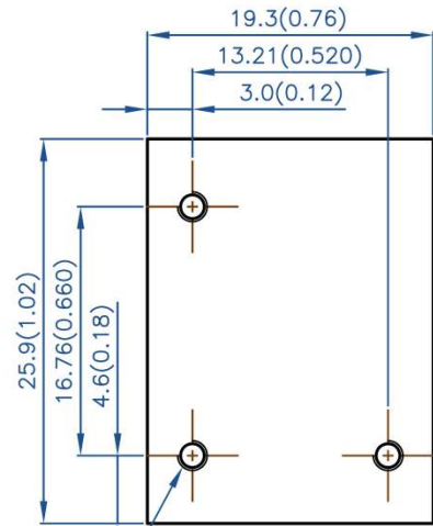
Baseplate Module
