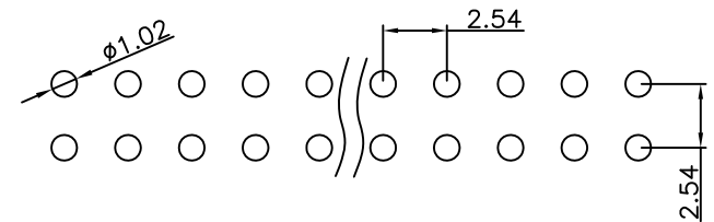
P.C.B LAYOUT
