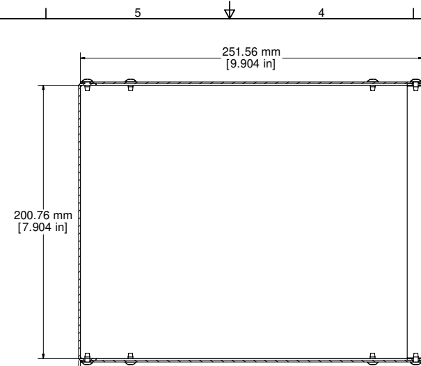
SECTION AA-AA
