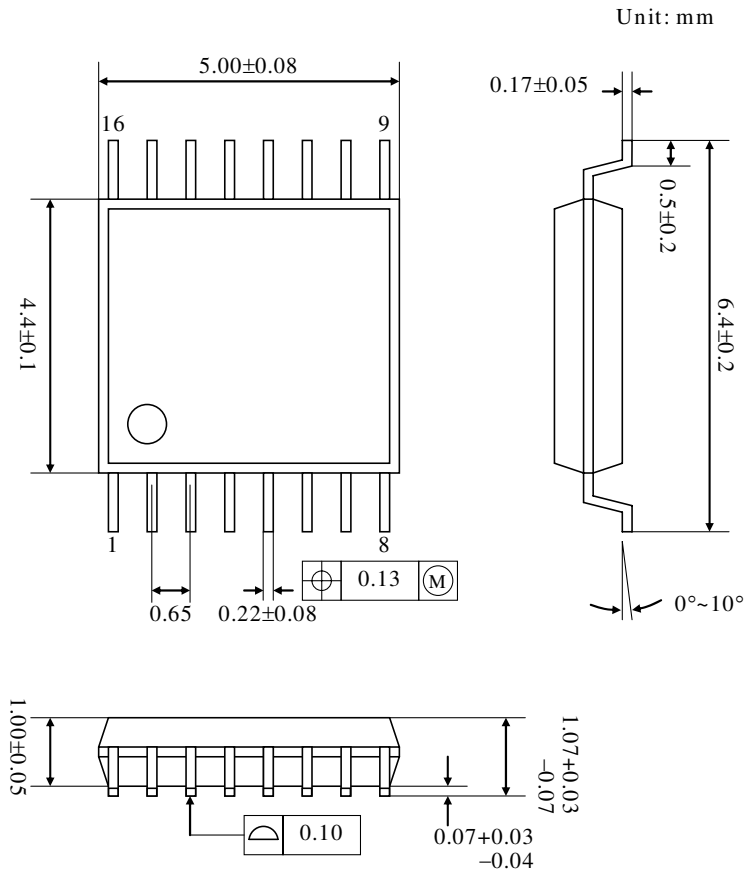
Fig. 30 Package dimensions
