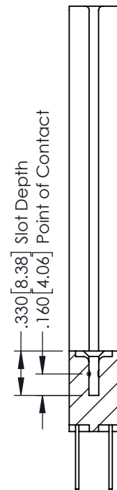
SECTION A-A
