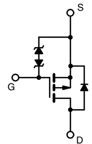
P-Channel MOSFET
