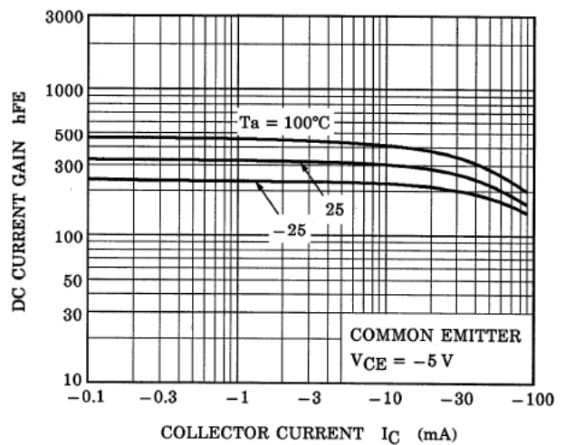
Fig. 9.6 RN2911EF h_{FE} - I_C
