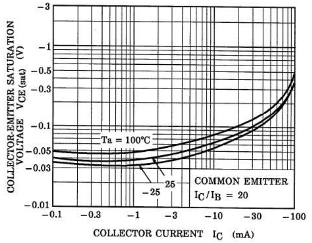
Fig. 9.8 RN2911EF V_{CE(sat)}-I_C
