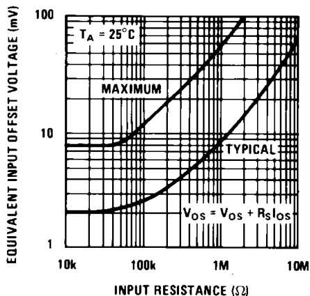
Offset Error
