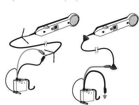
Figure 2a. Localisation d'une paire
