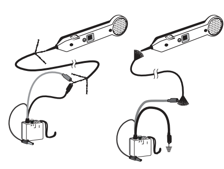
Figura 2a. Traccia della coppia
