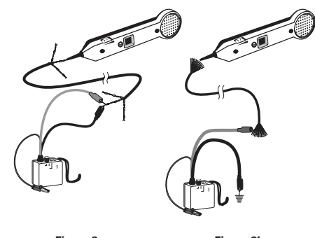
Figura 2a. Rastreo de pares
