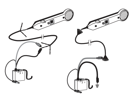
Figura 2a. Rastreamento de pares
