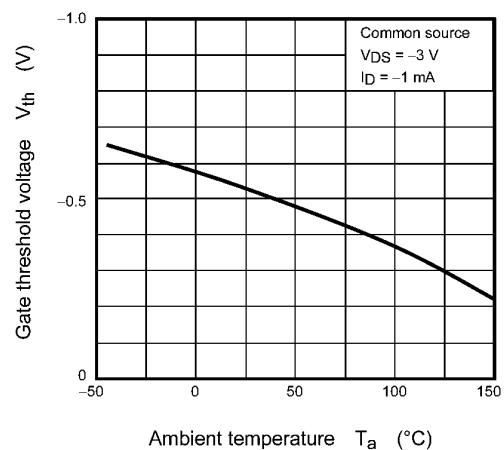
Fig. 7.6 V_{th} - T_A
