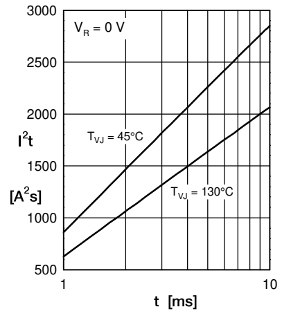
Fig. 3 I^2t vs. time per diode
