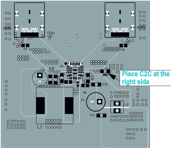
Top Layer
