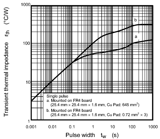
Fig. 7.12 r_{th} - t_w
