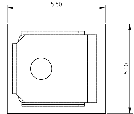
P.C.B LAYOUT:TOL±0.10
