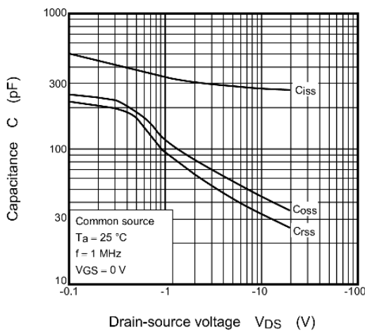
Fig. 7.9 C - V_{DS}
