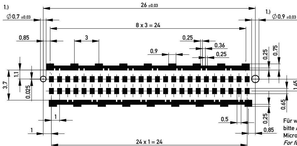
Leiterplatten-Layout Vorschlag / PCB-Layout Proposal
