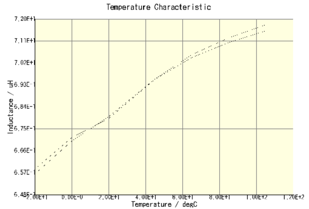
CLF10040T-680M-CA(DC = 0A)
