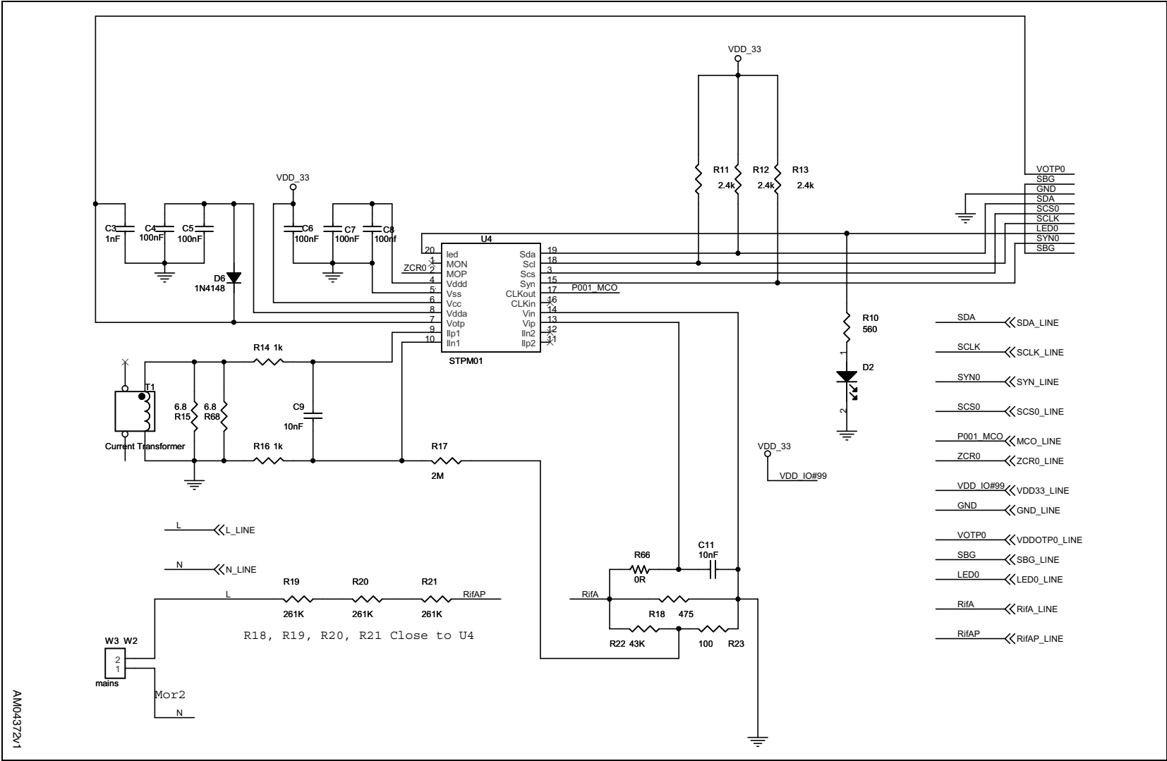
Figure 5. Energy meter IC
