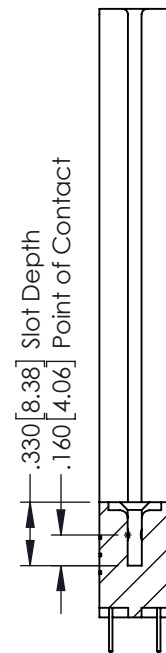
SECTION A-A
