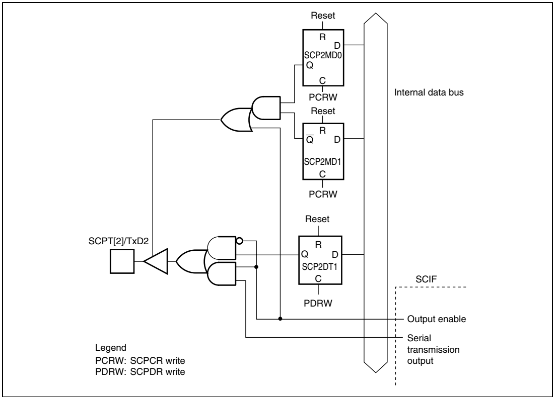
Figure 16.3 SCPT[2]/TxD2 Pin
