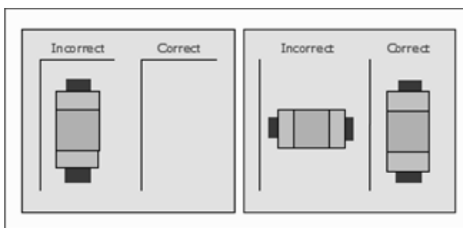
PCB Edge
