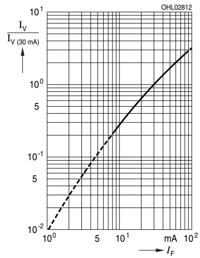
Relative Luminous Intensity 7) page 20, 8) page 20 Relative Lichtstärke 7) Seite 20, 8) Seite 20 I_V/I_V(30\text{ mA}) = f(I_F); T_S = 25^\circ\text{C}
