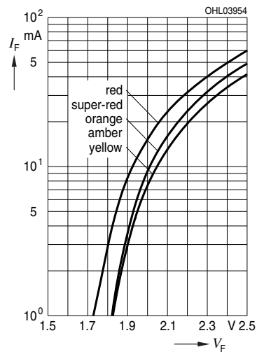
Forward Current 7) page 20 Durchlassstrom 7) Seite 20 I_F = f(V_F); T_S = 25^\circ\text{C}
