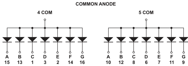
HDSP-G01E/G01G/G01Y/G01A
