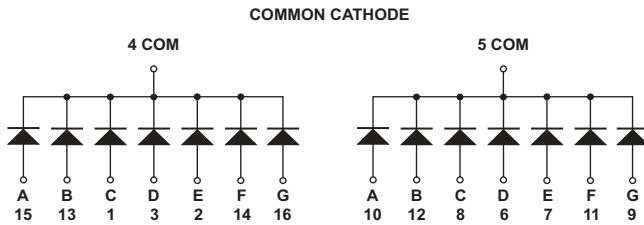
HDSP-G03E/G03G/G03Y/G03A
